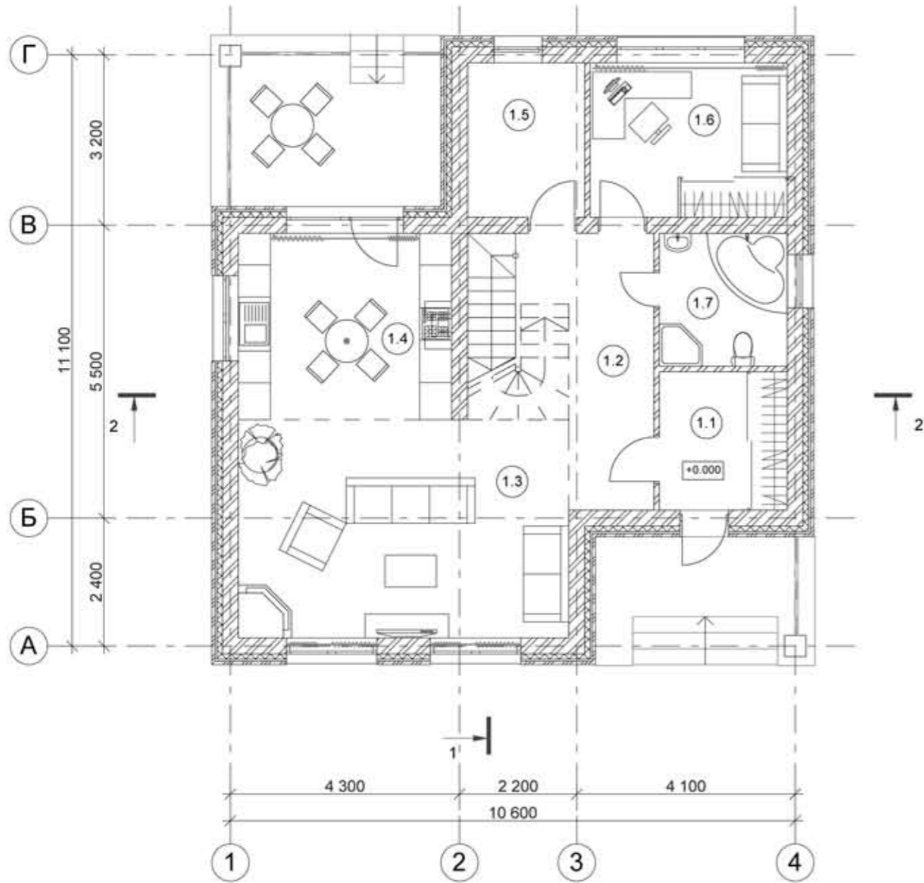
ПЛАН 1 ЭТАЖА
