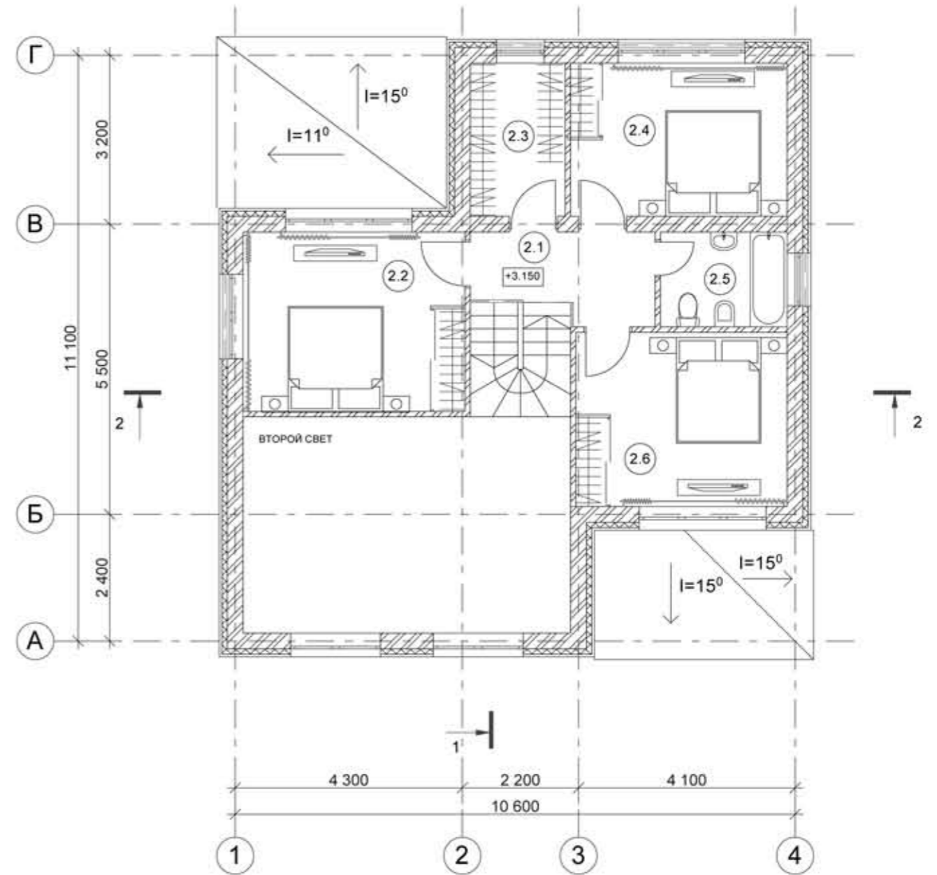
ПЛАН 2 ЭТАЖА
